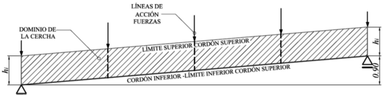
Fig. 4: Dominio geométrico.
