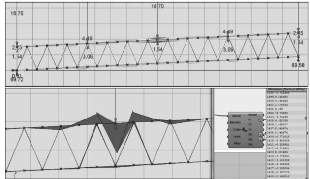
Fig. 8: Solicitación en barra debido a punto de aplicación de la carga.
