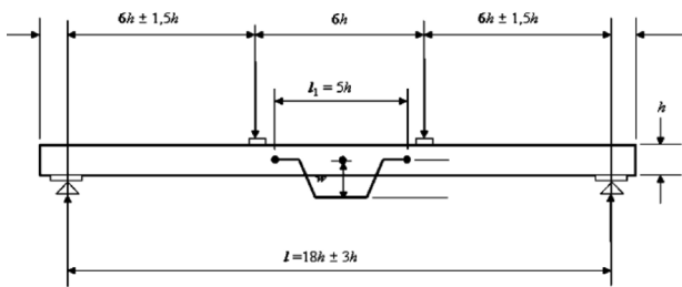
Fig. 1: Esquema general de carga del ensayo de flexión estática.
