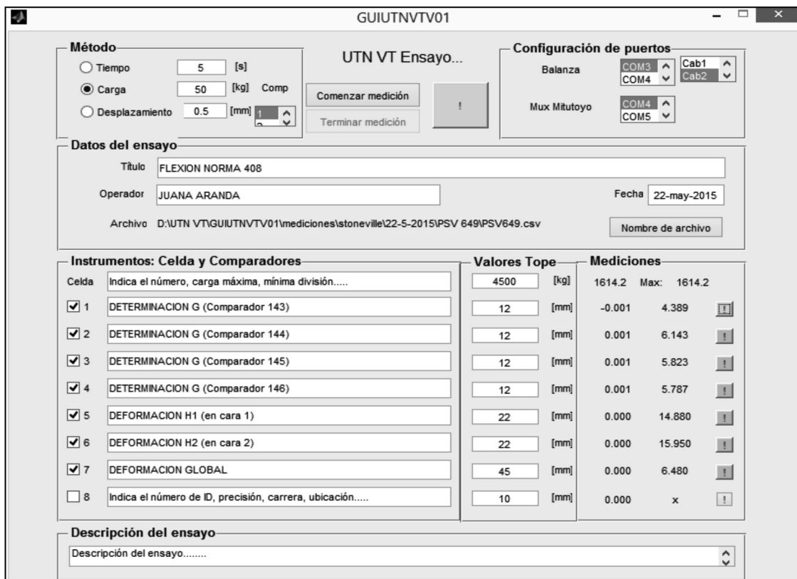
Fig. 7: Interface de usuario.
