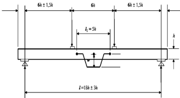
Fig. 1: Esquema de carga.
