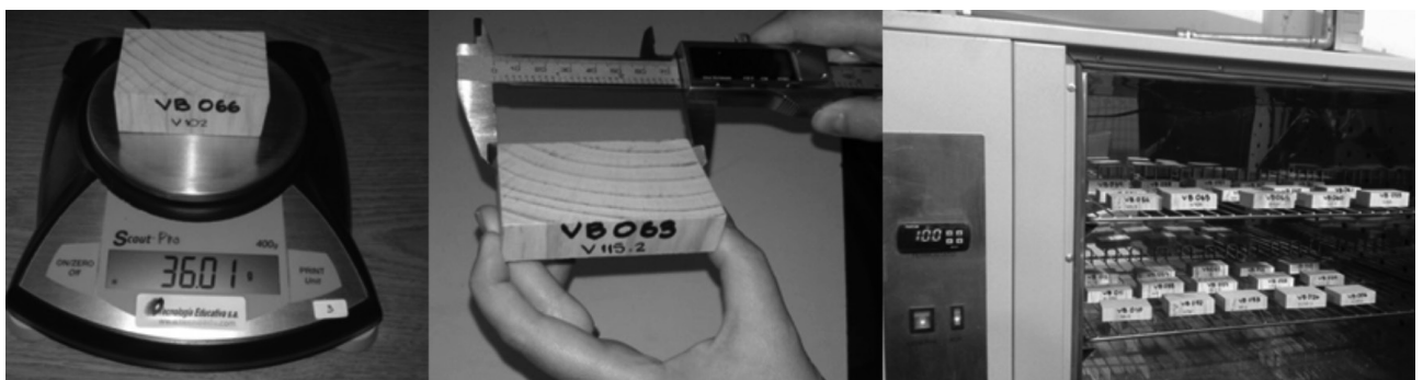
Fig. 3: Pesado - Cubicado - Secado en Horno.
