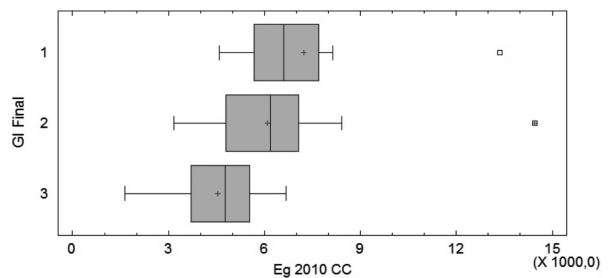
Gráfico 2: Análisis estadístico del Módulo de Elasticidad.
