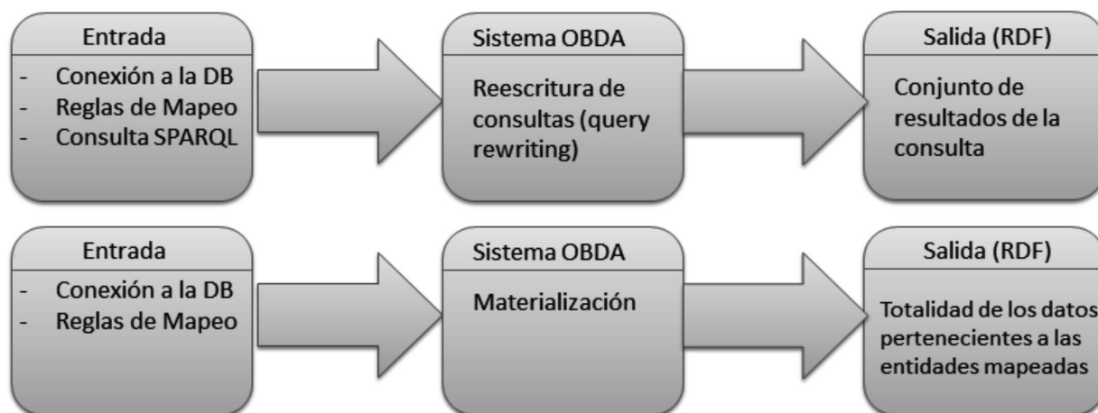
Fig. 1: Distintas metodologías de OBDA.
