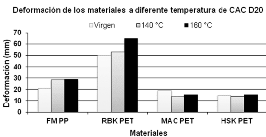
FIGURA 10. DEFORMACIÓN DE LOS MATERIALES GEOSINTÉTICOS ANTES Y DESPUÉS DE SER SOMETIDOS A TEMPERATURA.
