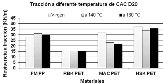
FIGURA 9. RESISTENCIA A TRACCIÓN DE LOS MATERIALES GEOSINTÉTICOS ANTES Y DESPUÉS DE SER SOMETIDOS A TEMPERATURA.
