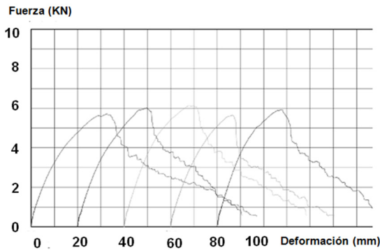
FIG. 16. FM PP LUEGO DE SOMETERLO A 160 °C DE MEZCLA ASFÁLTICA CONVENCIONAL.
