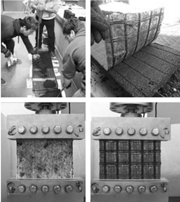
FIGURA 7. RECUPERACIÓN Y ENSAYO DE TRACCIÓN DE LA MUESTRA LUEGO DE SER SOMETIDA A MEZCLA ASFÁLTICA A TEMPERATURAS DE 140 °C Y 160 °C.
