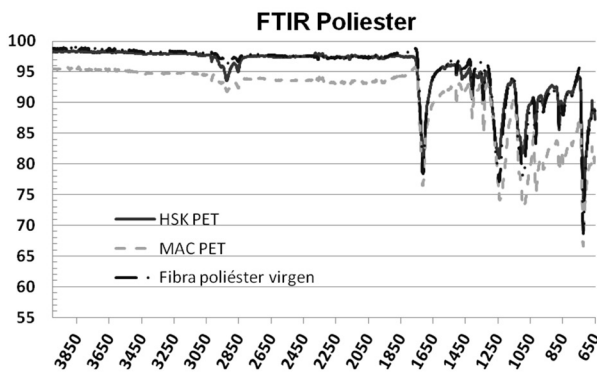
FIGURA 6. ESPECTRO IR DEL POLIÉSTER.
