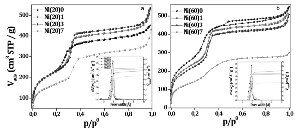
Figura 3. Isothermas de adsorción-desorción de N 2 a 77 K de las muestras con relación Si/Ni a) 20 y b) 60. Inset DTP de los materiales estudiados.
