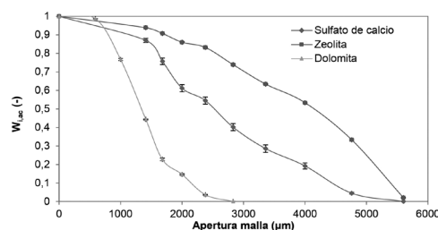
Figura 2. Distribución de tamaño de partículas para los diferentes núcleos.
