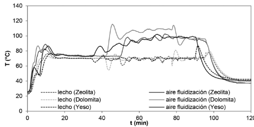
Figura 5. Segundo recubrimiento de los tres materiales con T_{lecho}^{SP} = 70\text{ }^{\circ}\text{C} .
