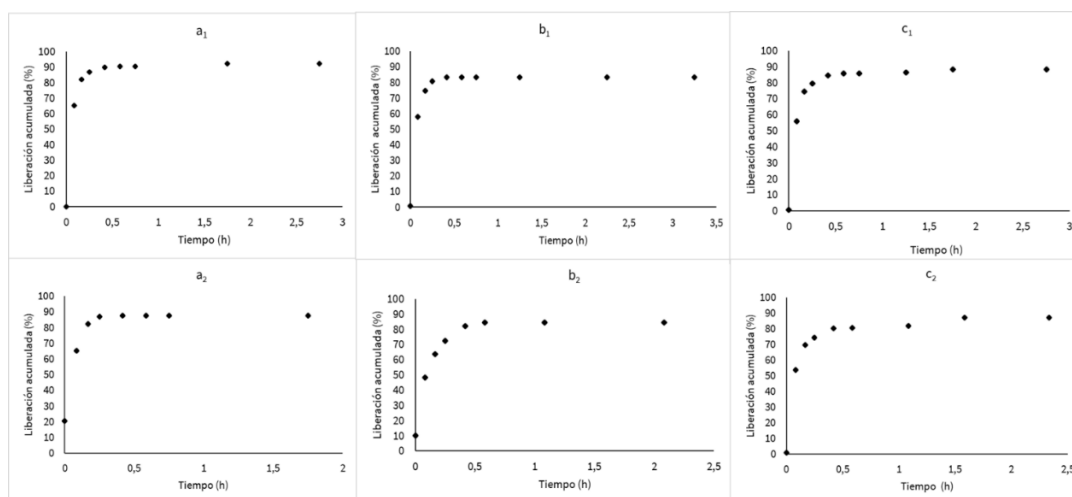
Figura 3: Liberación controlada de microcápsulas húmedas sin sólido ( a_1 ), con sílice ( b_1 ) y con almidón ( c_1 ); y de microcápsulas con secado sin sólido ( a_2 ), con almidón ( b_2 ) y con sílice ( c_2 )
