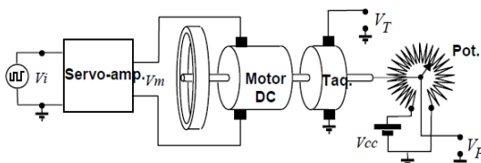
Fig.2: Esquema del sistema de control de posición a lazo abierto
