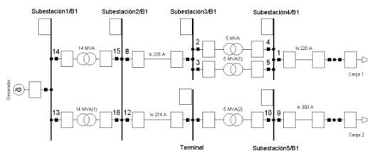
Fig. 7. Red propuesta.
