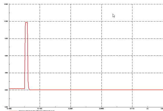
Fig. 6. Simulación de corto circuito (valores RMS).
