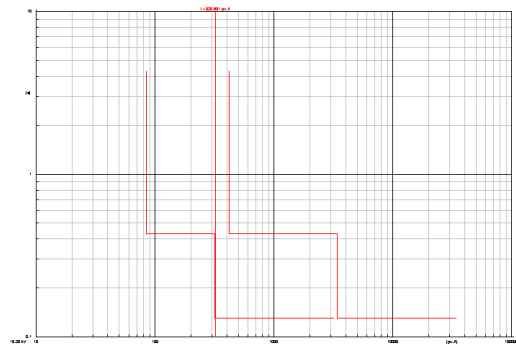
Fig. 8. Diagramas tiempo-corriente del relé 9 (red propuesta).
