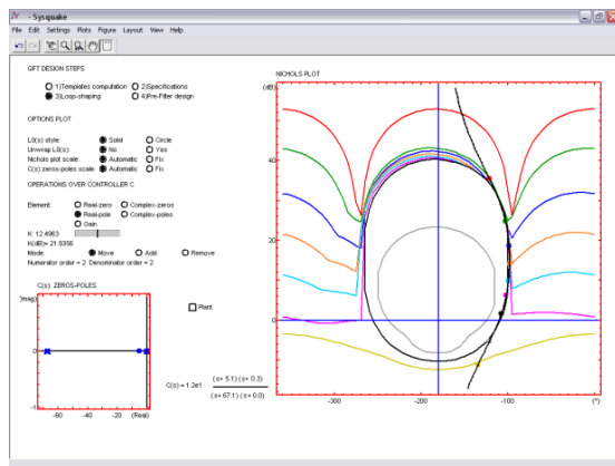
Fig. 3: Herramienta de CAD: SISO QFTIT- Ventana de diseño del controlador
