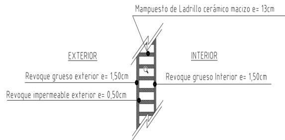
Figura 2: Propuesta de envolvente número 2.
