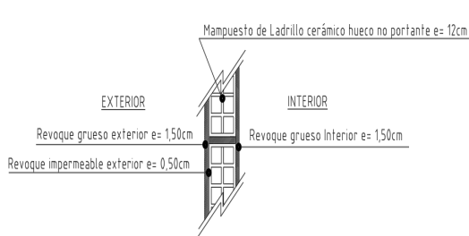
Figura 1: Propuesta de envolvente número 1.
