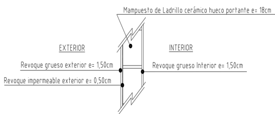
Figura 3: Propuesta de envolvente número 3.
